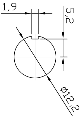
安装面板尺寸 PANEL CUT-OUT
